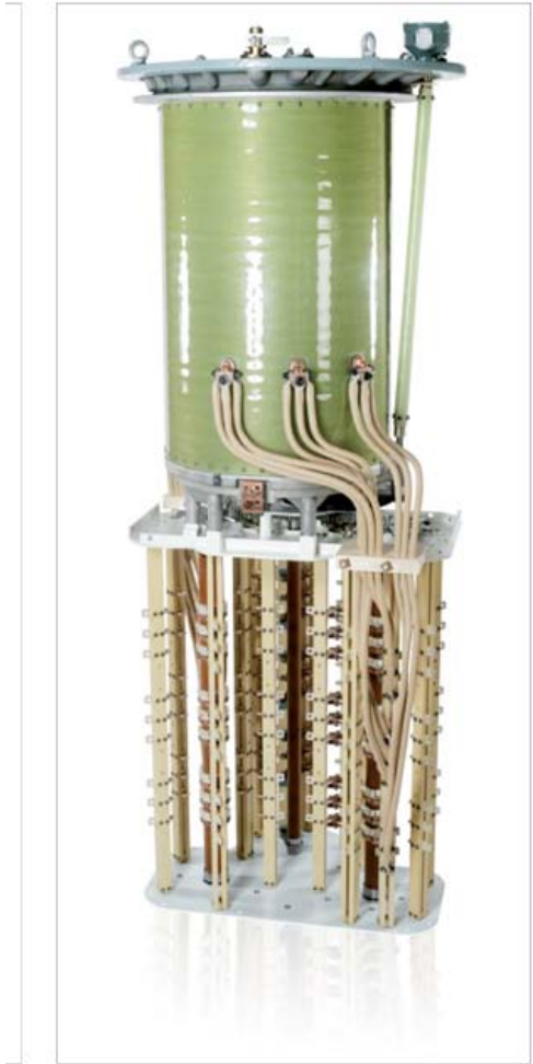
On-load tap-changer, type UCC
